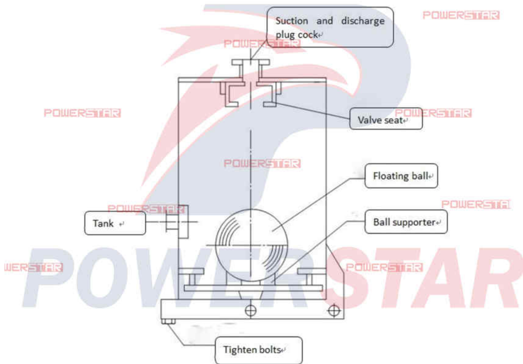
(Water-Gas Separator)
